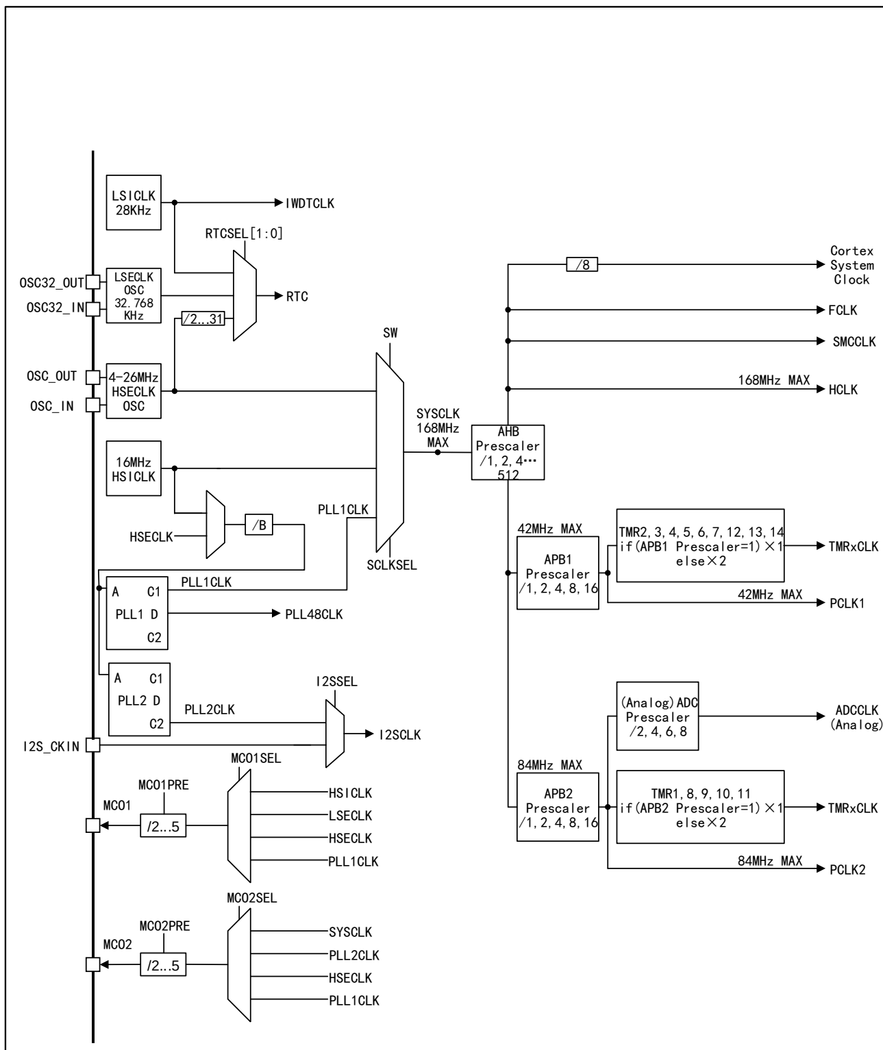
图 6 APM32F465xE 时钟树
