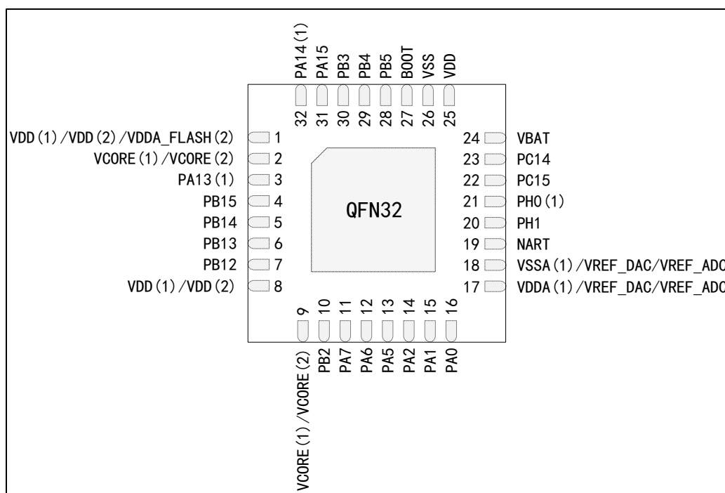
图 4 APM32F465xE 系列 QF32 引脚分布图
