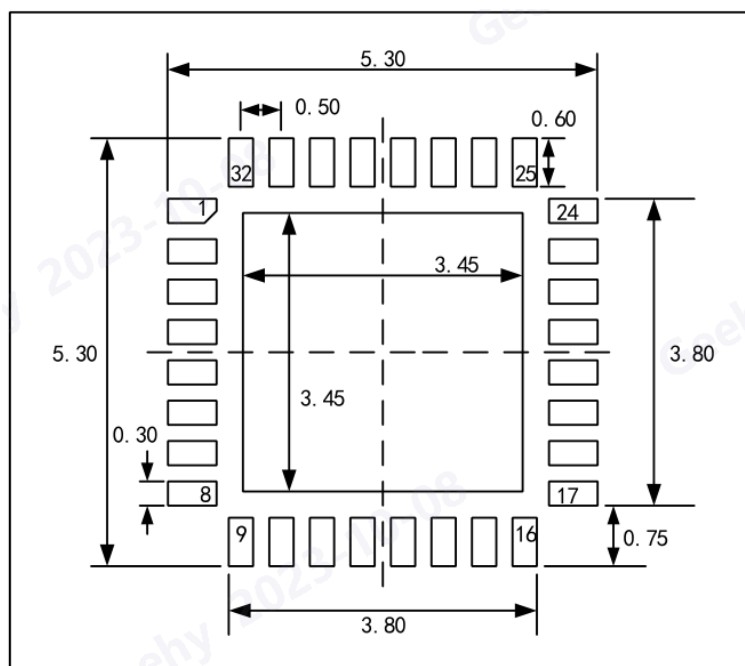
图 32 QFN32 焊接 Layout 建议
