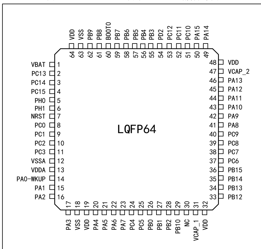
图 2 APM32F465xE 系列 LQFP64 引脚分布图
