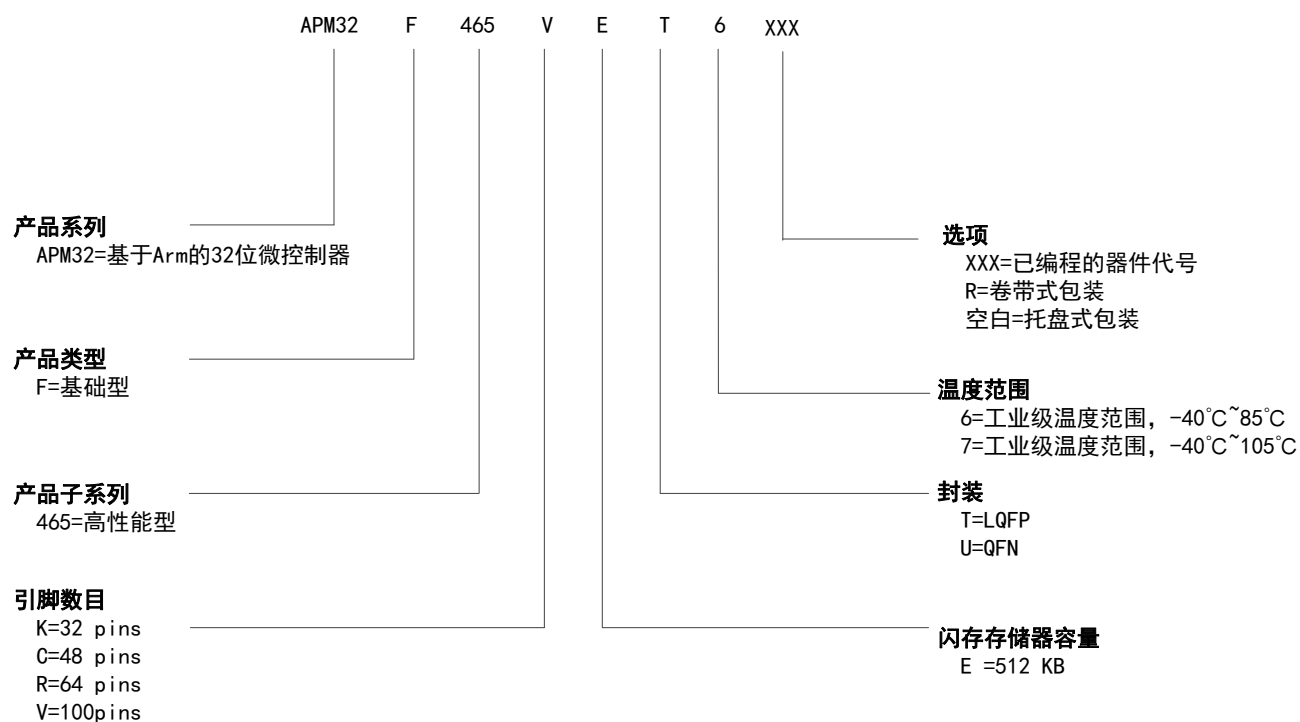
图 27 APM32F465xE 系列订货信息图
