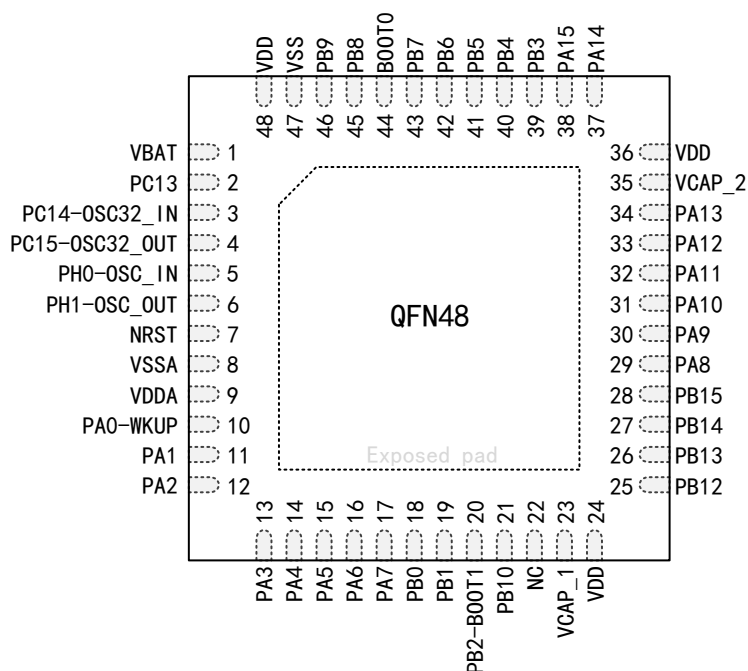
图 3 APM32F465xE 系列 QFN48 引脚分布图
