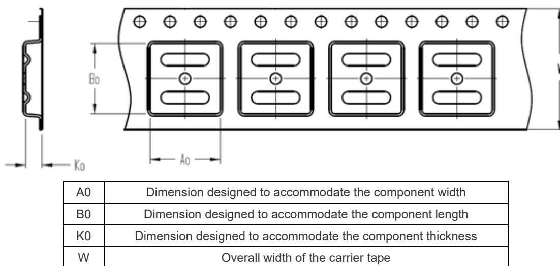
图 25 带状包装规格图
