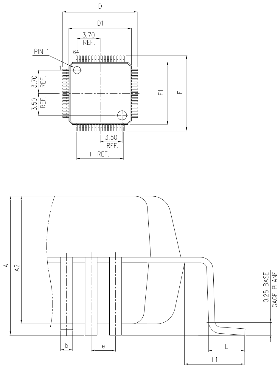
图 19 LQFP64 封装图
