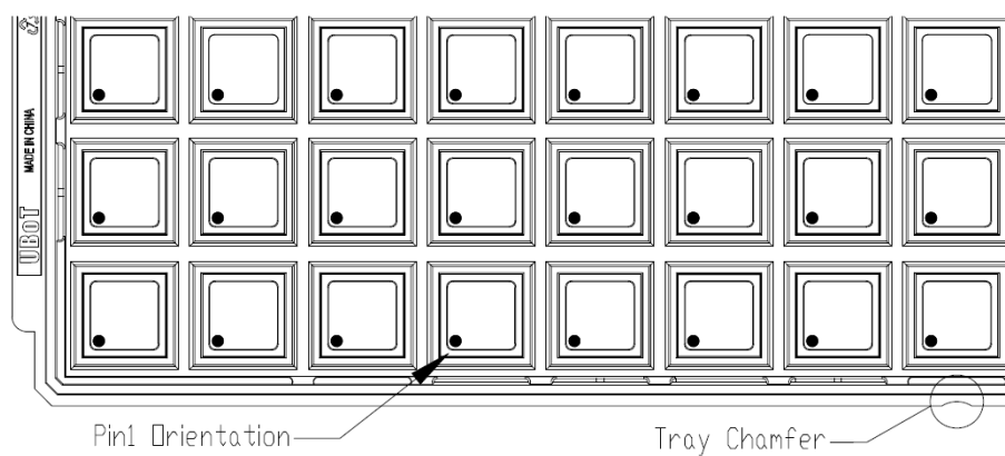
图 26 托盘包装示意图
