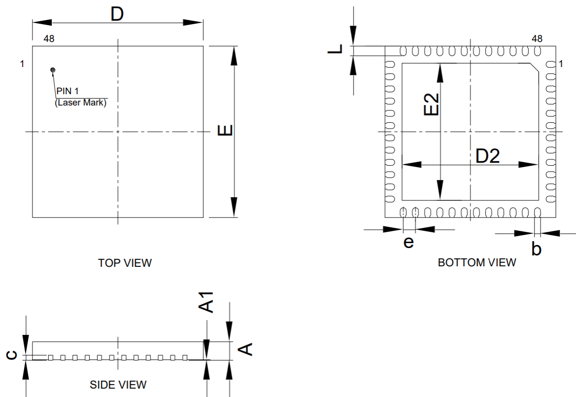
图 22 QFN48 封装图
