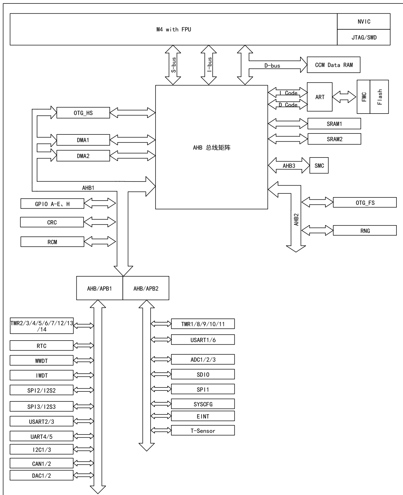
图 5 APM32F465xE 系统框图
