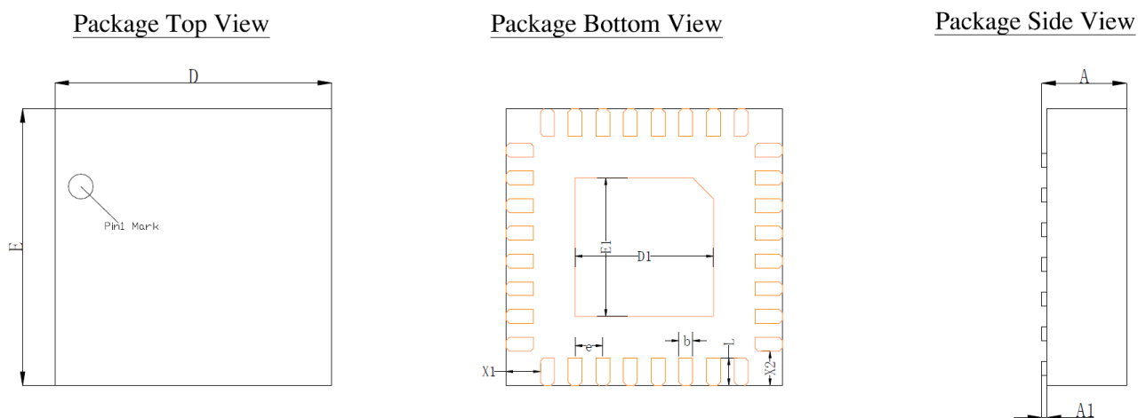
图 31 QFN32 封装图
